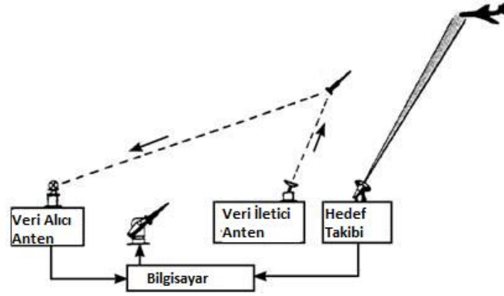
Şekil 18: Komut G d m Sistemi  alıřma Prensibi [15]
