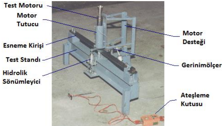
Şekil 39: Dikey Test Düzeneği [2]
