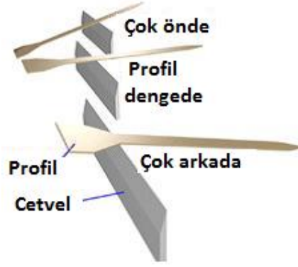
Şekil 43: Roket Profili Kullanarak Basınç Merkezinin Bulunması [3]
