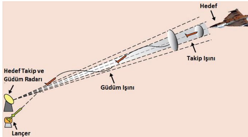
Şekil 21: Radar Kullanılarak Yapılan Işın İzleme Güdüm Sistemi [18]
