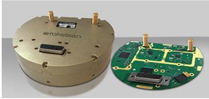
Şekil 20: Roketsan Tarafından Tasarlanan KKS Alıcısı
