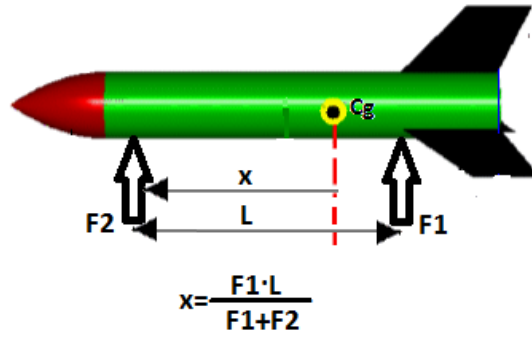
Şekil 41: Yük Hücreleri ile Ağırlık Merkezinin Bulunması [4]
