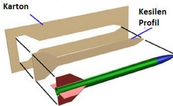
Şekil 42: Basınç Merkezinin Bulunabilmesi için Profil Çıkartılması [3]
