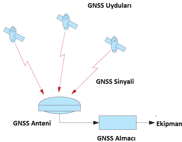
Şekil 19: GNSS  alıřma Prensibi [17]
