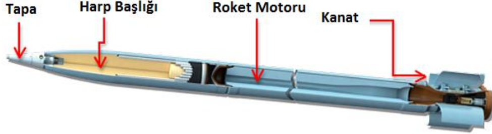
Şekil 2: 122mm Roketin Bölümleri [2]
