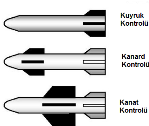
Şekil 6: Füzelerde Kontrol Tipleri [6]
