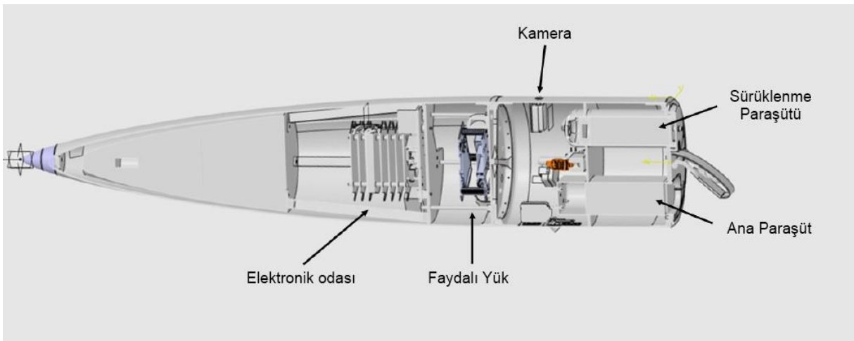
Şekil 30: Stratos III Burun Kesiti
