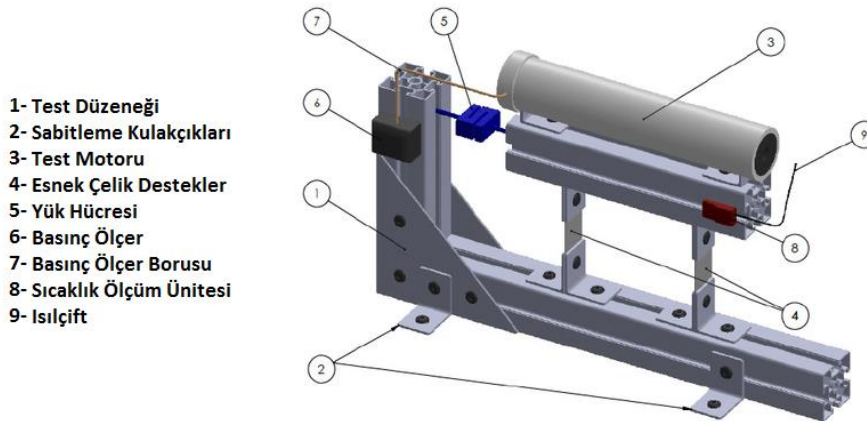
Şekil 38: Yatay Test Düzeneği [1]
