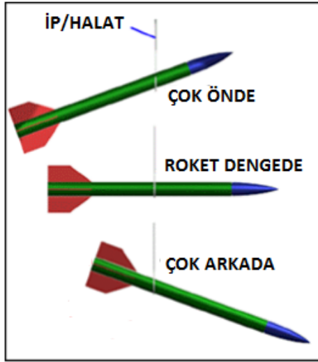
Şekil 40: Ağırlık Merkezinin İp Yardımıyla Bulunması [3]
