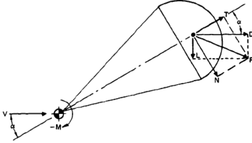
Şekil 31: Paraşüt Üzerindeki Kuvvetler
