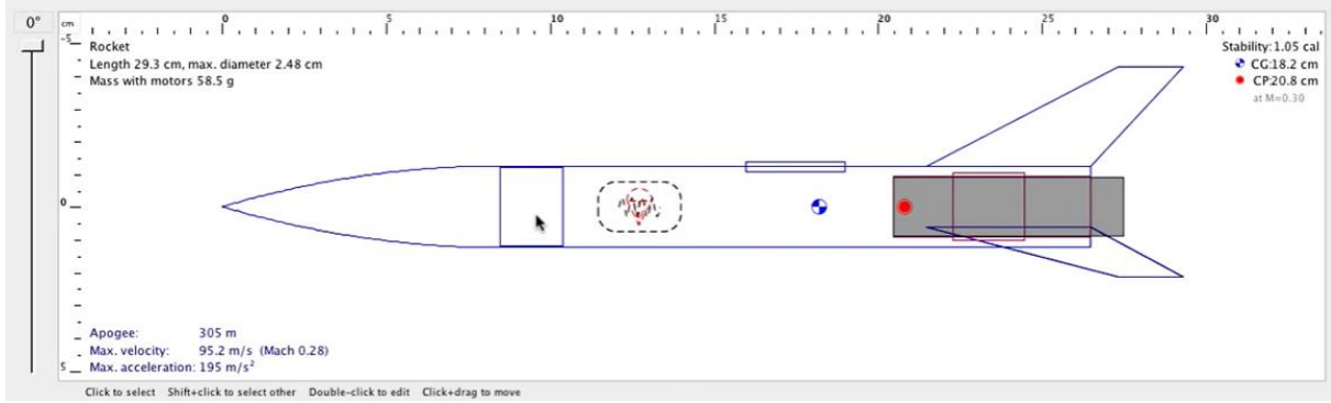
Şekil 44: OpenRocket Yazılımı Kullanılarak CG ve Cp'nin Bulunması
