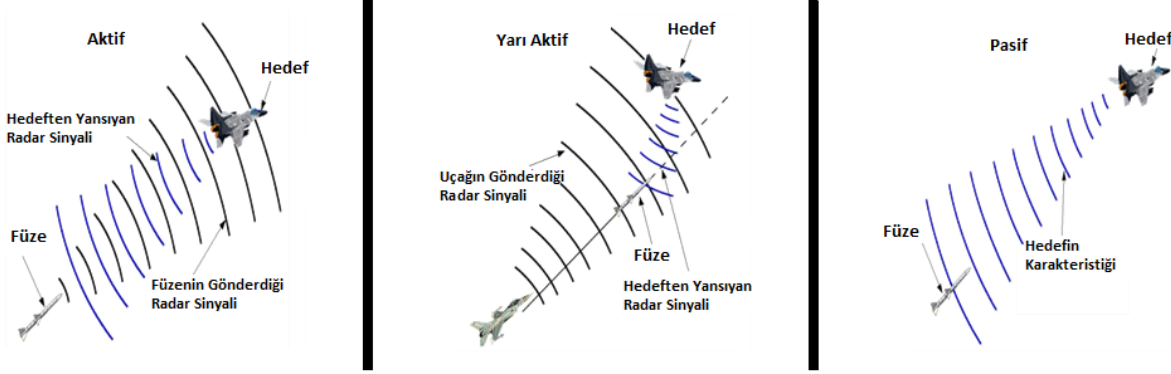
Şekil 17: Arayıcı Başlıklı Güdümlü Sistemi Tipleri [13]
