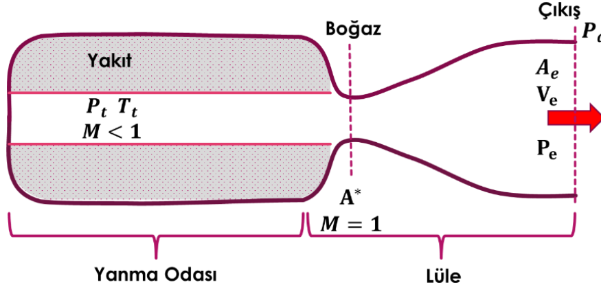
Şekil 23: Yanma Odası Şematik Gösterimi
