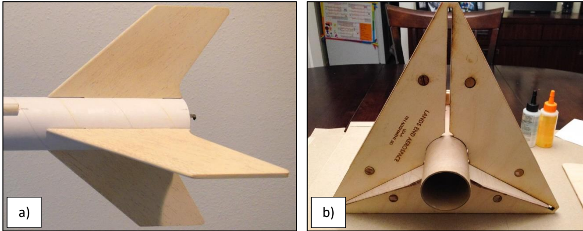
Şekil 34: a) Balsa Kanat Örneği [3] b) Kanat Hizalama Aparatı Örneği [4]
