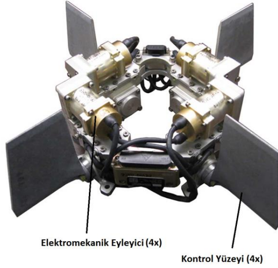
Şekil 9: Elektromekanik Eyleyici [7]
