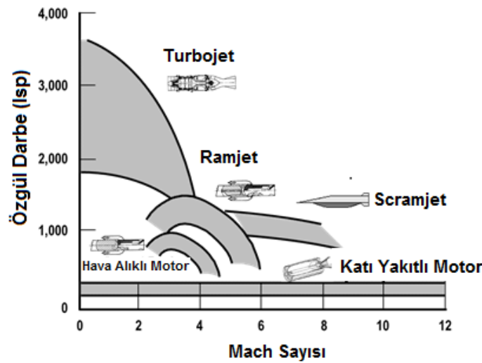
Şekil 13: Farklı İtki Sistemlerinin Özgül Darbelerinin Mach Sayısı ile Değişimi [10]
