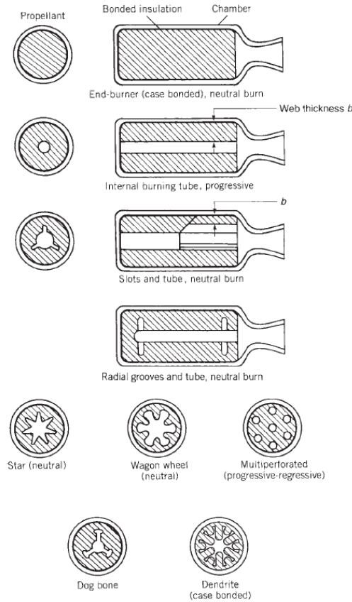
Şekil 25: Katı Yakıt Profil Örnekleri
