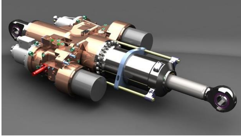
Şekil 10: Elektrohidrolik Eyleyici [8]
